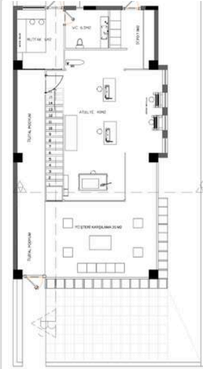
Zemin Kat Planı 1/50
