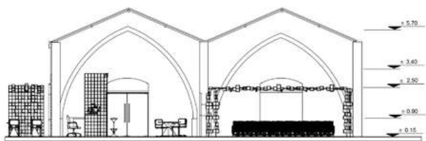
B'-B' KESİT ÖLÇEK:1/50
