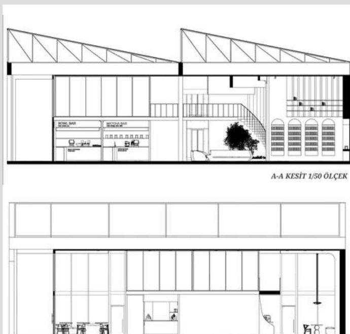
Kesit
