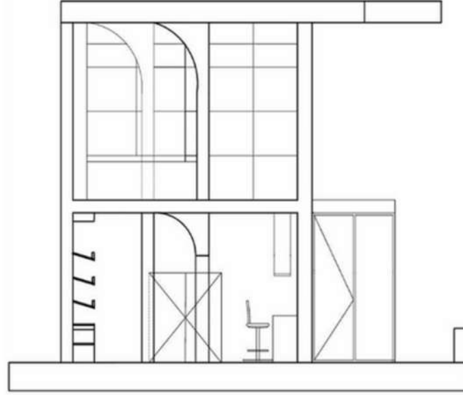
Görünüş
