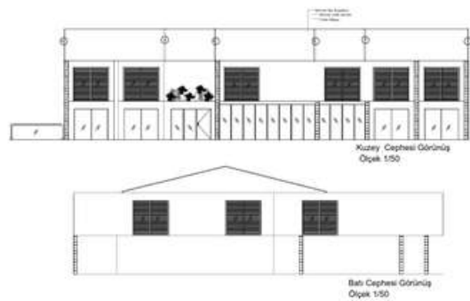
Görünüş
