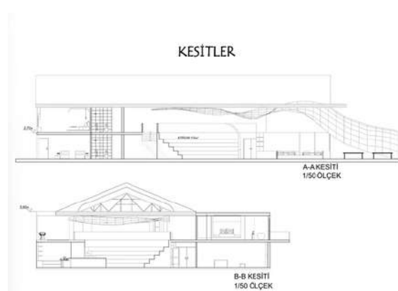
Kesit
