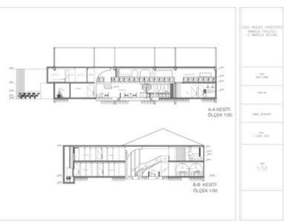
Kesit
