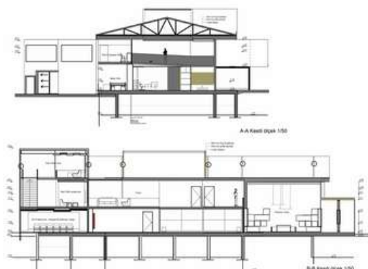
Kesit
