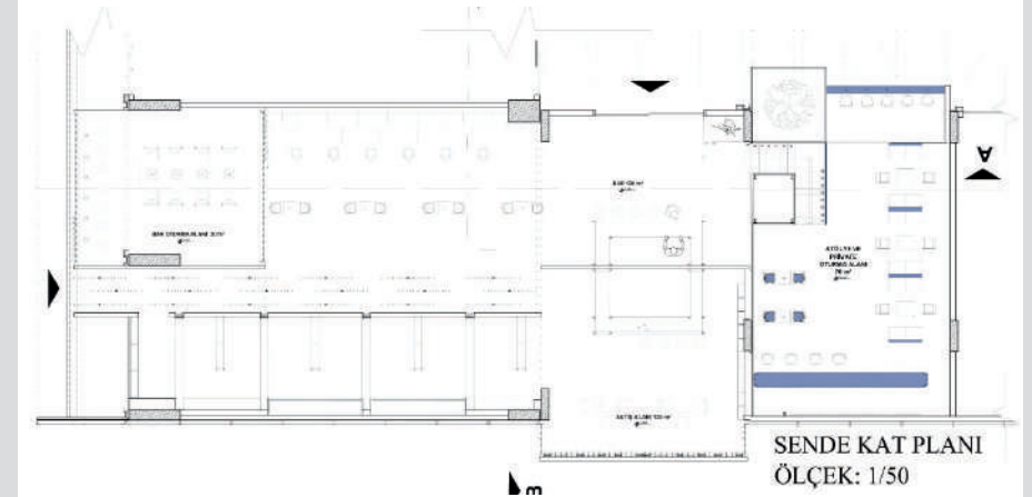
ZEMİN KAT PLANI ÖLÇEK: 1/50
